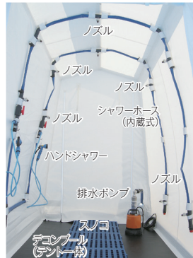
MQ-DTS-2 内観
