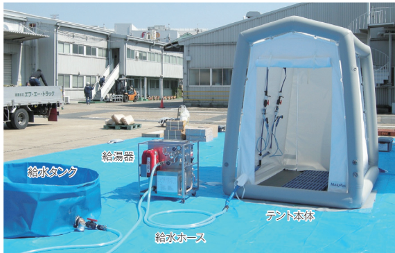
MQ-DTS-2 外観・配置例
